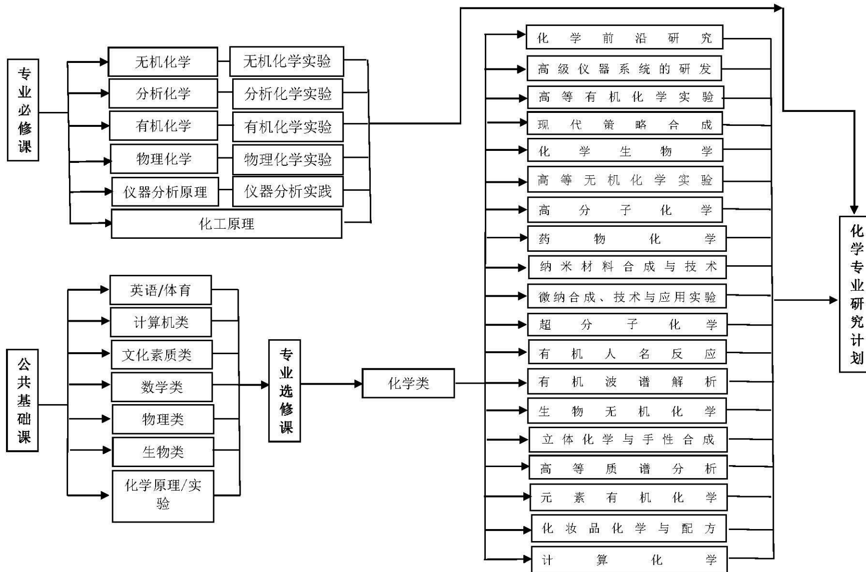
化学专业主要课程关系图
